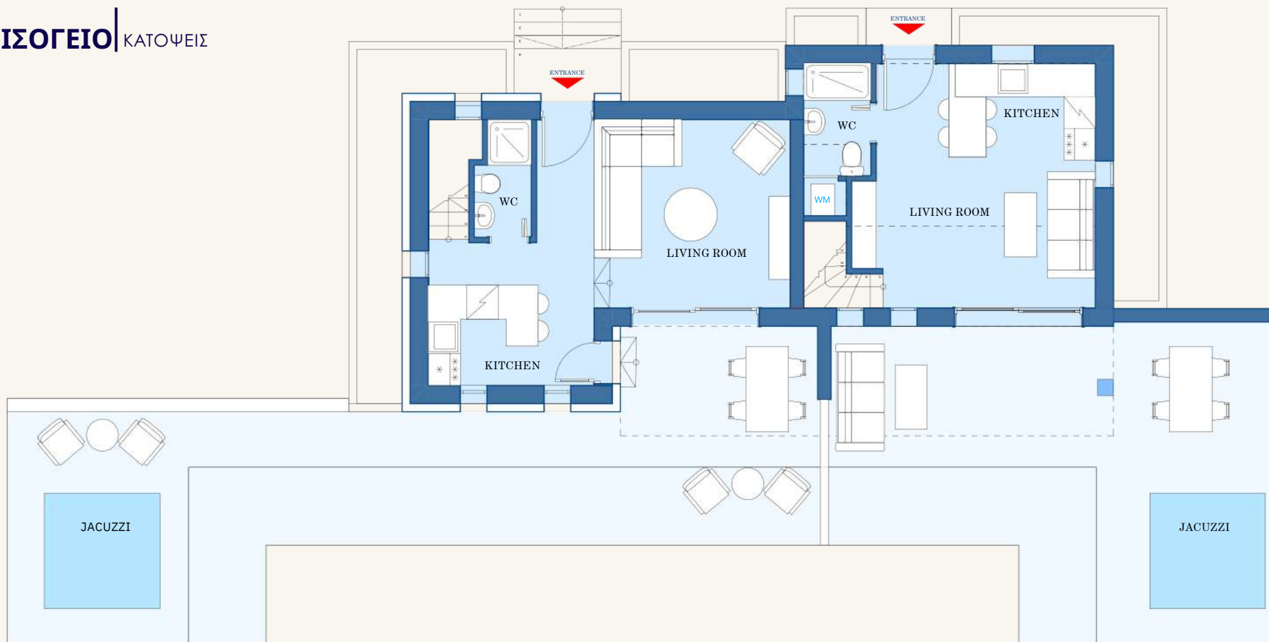
ΤΥΠΙΚΗ ΚΑΤΟΨΗ ΙΣΟΓΕΙΟΥ ΕΠΙΦΑΝΕΙΑ ΚΑΤΟΙΚΙΑΣ ΤΥΠΟΥ Α
